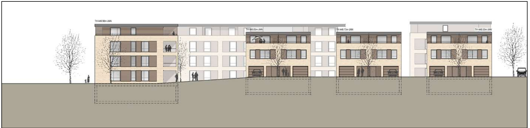
Ansicht Nord
